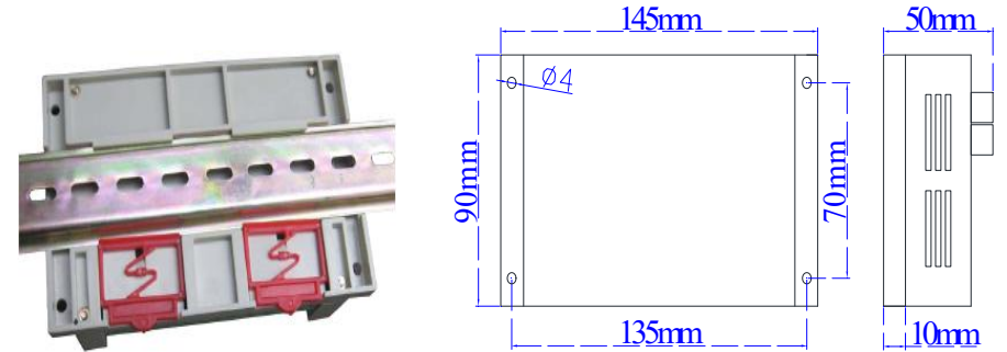
35mm DIN 导轨安装
