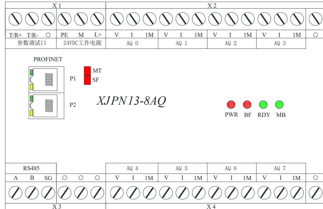
35mm DIN 导轨安装
